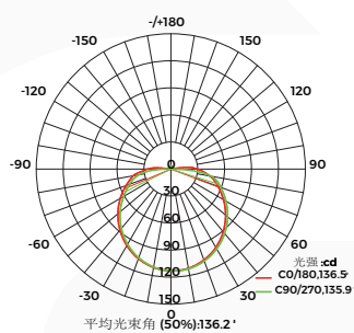
· 配光曲线图
